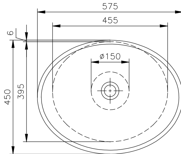
LAVABO SOFT ( SIN REPISA )
