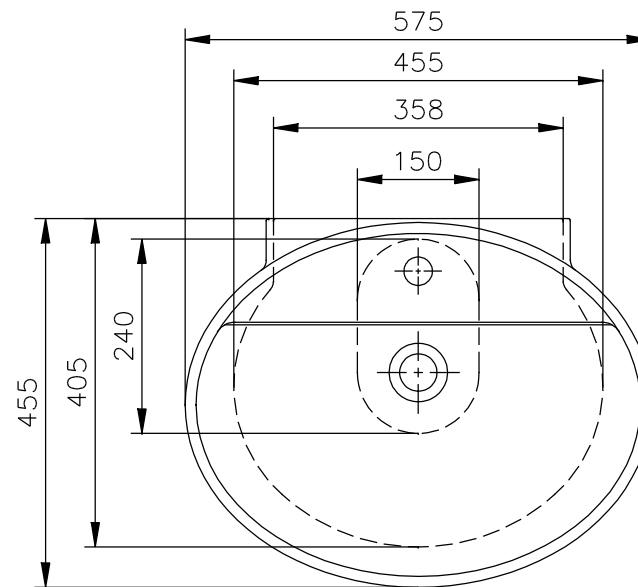
LAVABO SOFT ( CON REPISA )
