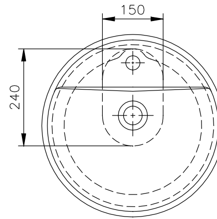
LAVABO URBAN-45 ( CON REPISA )
